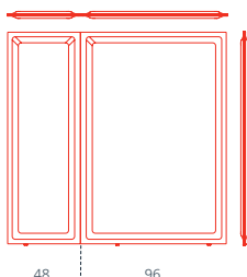
Acoustic panel H140 1ML0140 L 144 P 4,6 H 140
